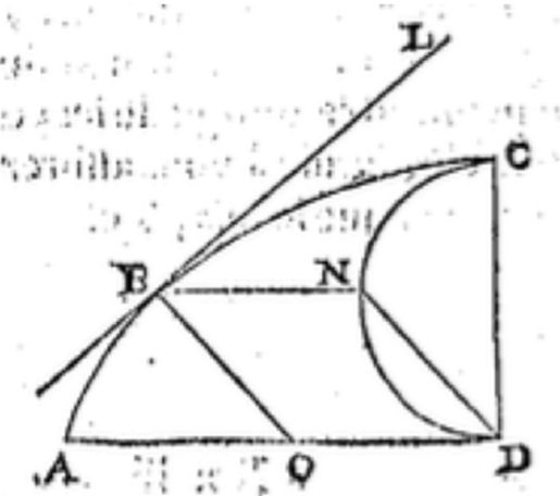
Εικόνα 4: Η ίδια ερώτηση απαντήθηκε από τον Καρτέσιο το 1638: το σημείο O της επαφής του ακίνητου κύκλου είναι στιγμιαίο κέντρο περιστροφής, και επομένως η εφαπτομένη BL είναι κάθετη στην BO, κάτι που στη συνέχεια οδηγεί στο γεγονός ότι η BL είναι παράλληλη με την NC.
